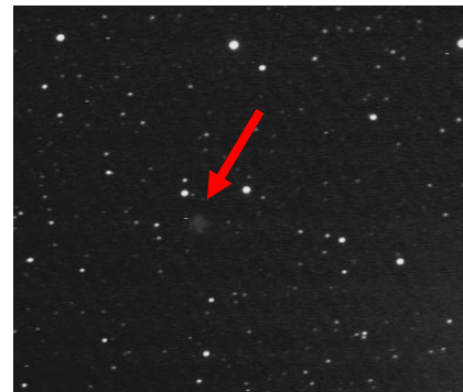
M2-55 - Cepheus
