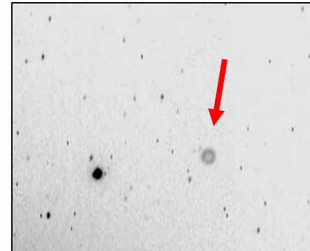
Abell-81 - Cepheus
