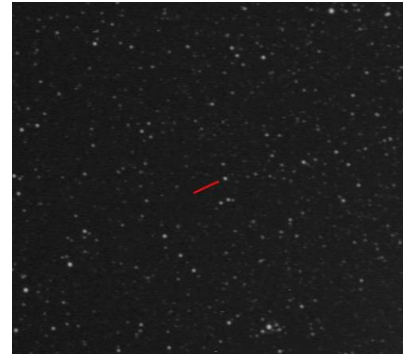
M1-59 - Scutum
