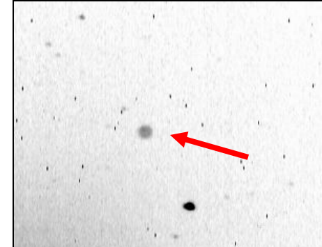
Abell-50 - Draco
